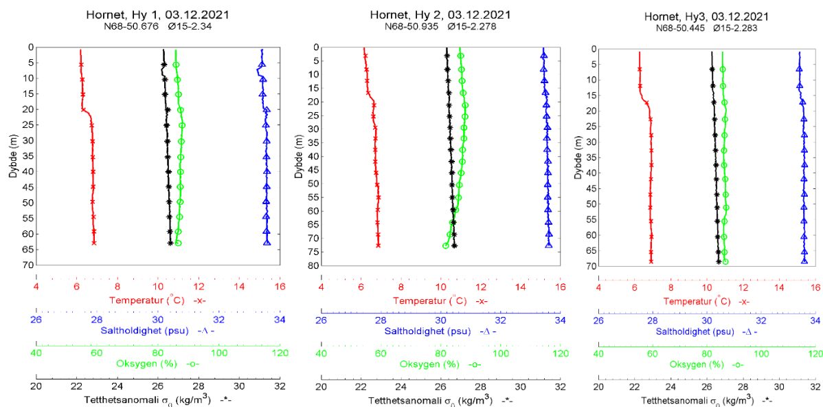
Figur 3. Vertikalprofiler for temperatur, saltholdighet, tetthet og oksygennivåer fra overflate til bunn på stasjonene Hy1, Hy2 og Hy3 den 03.12.2021.
