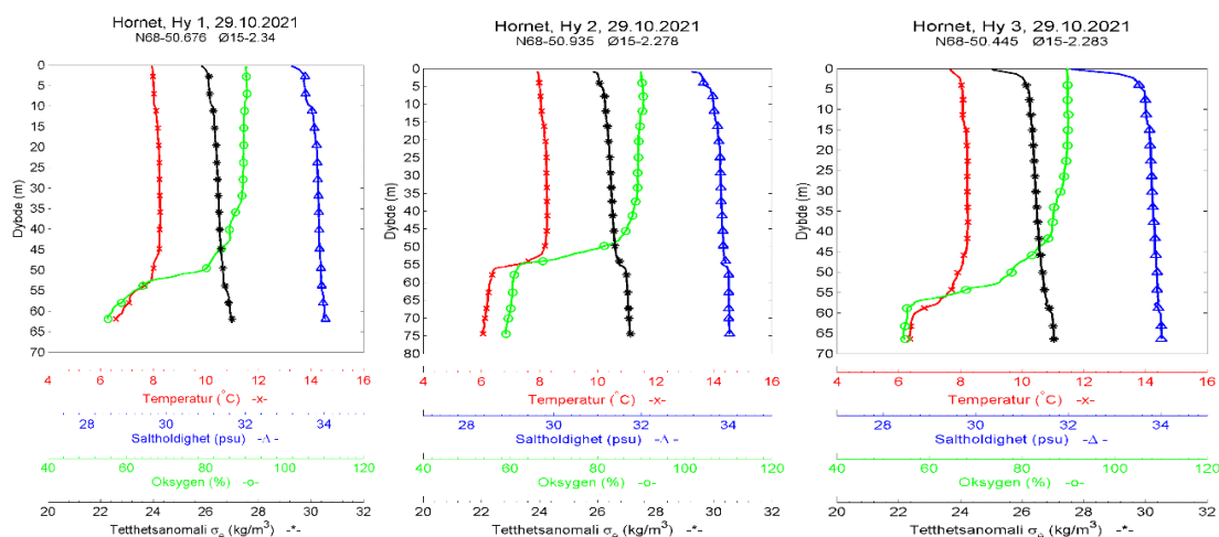
Figur 2. Vertikalprofiler for temperatur, saltholdighet, tetthet og oksygennivåer fra overflate til bunn på stasjonene Hy1, Hy2 og Hy3 den 29.10.2021.
